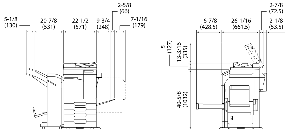
Основной блок + DF-633 + PC-218 + FS-539 SD + RU-514 + МК-711 + Д-101 Единица измерения: дюйм (мм)
